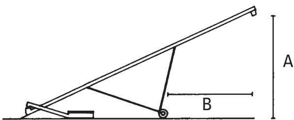
Mått på MK skruvar ▼
